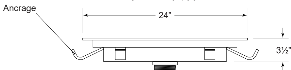
VUE DE FACE/COTÉ
