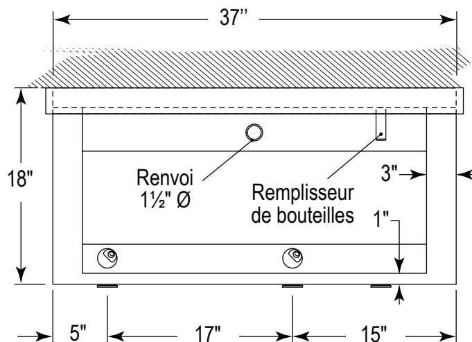
VUE DE DESSUS (Modèle illustré: 2 stations avec option RB)
