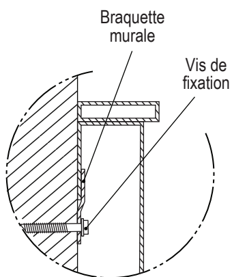
DÉTAIL C
