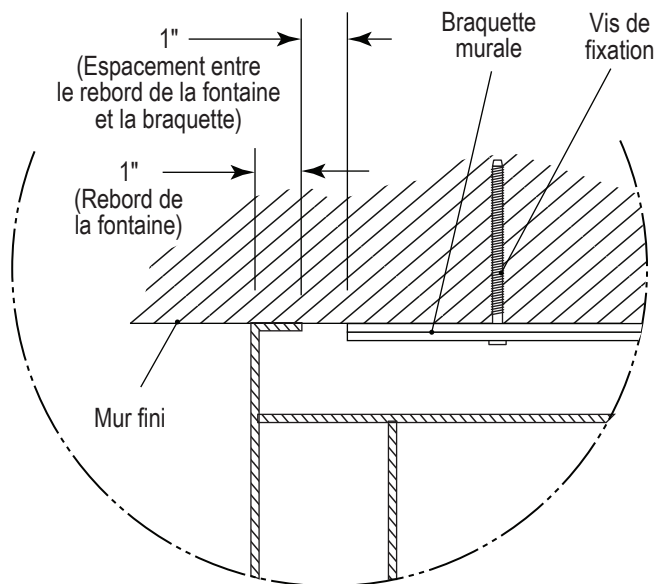
DÉTAIL B
